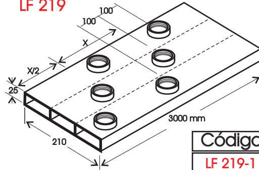
Duto Modulado Paralelo 3x25x70 mm
