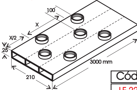
Duto Modulado Alternado 3x25x70 mm
