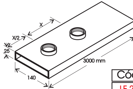
Duto Modulado 25x140 mm
