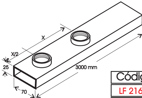
Duto Modulado 25x70 mm
