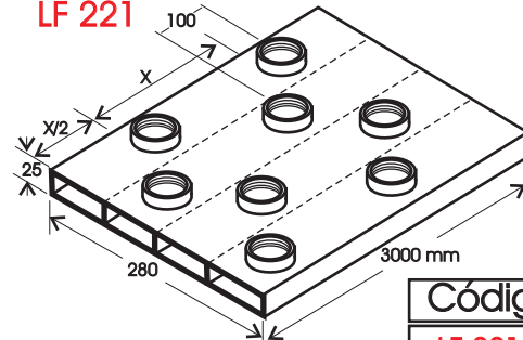
Duto Modulado Alternado 4x25x70 mm
