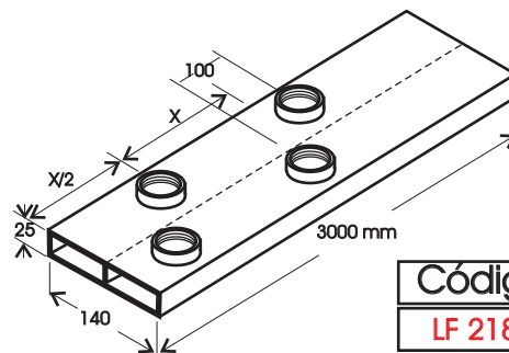
Duto Modulado 2x25x70 mm
