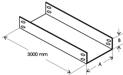
Eletrocalha Lisa LF 110
