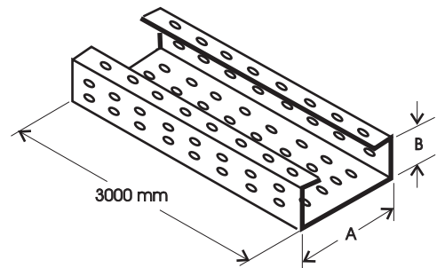
Eletrocalha Perfurada com Virola LF 113
